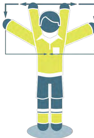
“ТВ” сигнал
